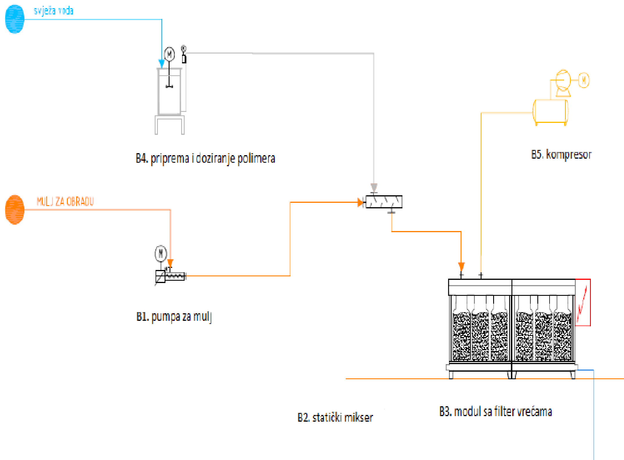
SHEMA DEHIDRACIJE MULJA
